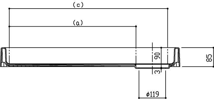
断面A-A
